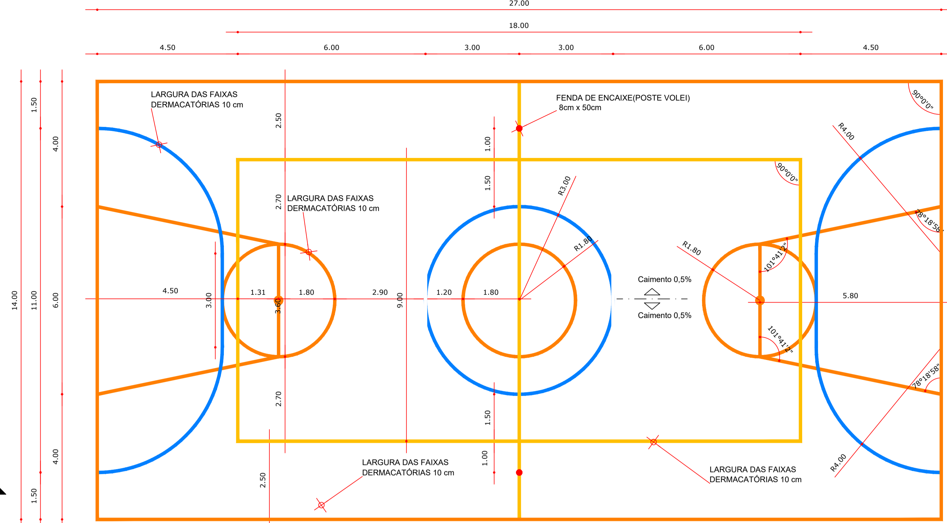
PINTURA DO PISO DA QUADRA - FAIXAS ESCALA 1:75
