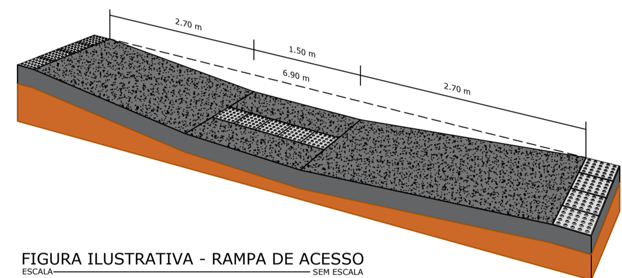
FIGURA ILUSTRATIVA - RAMPA DE ACESSO ESCALA SEM ESCALA
