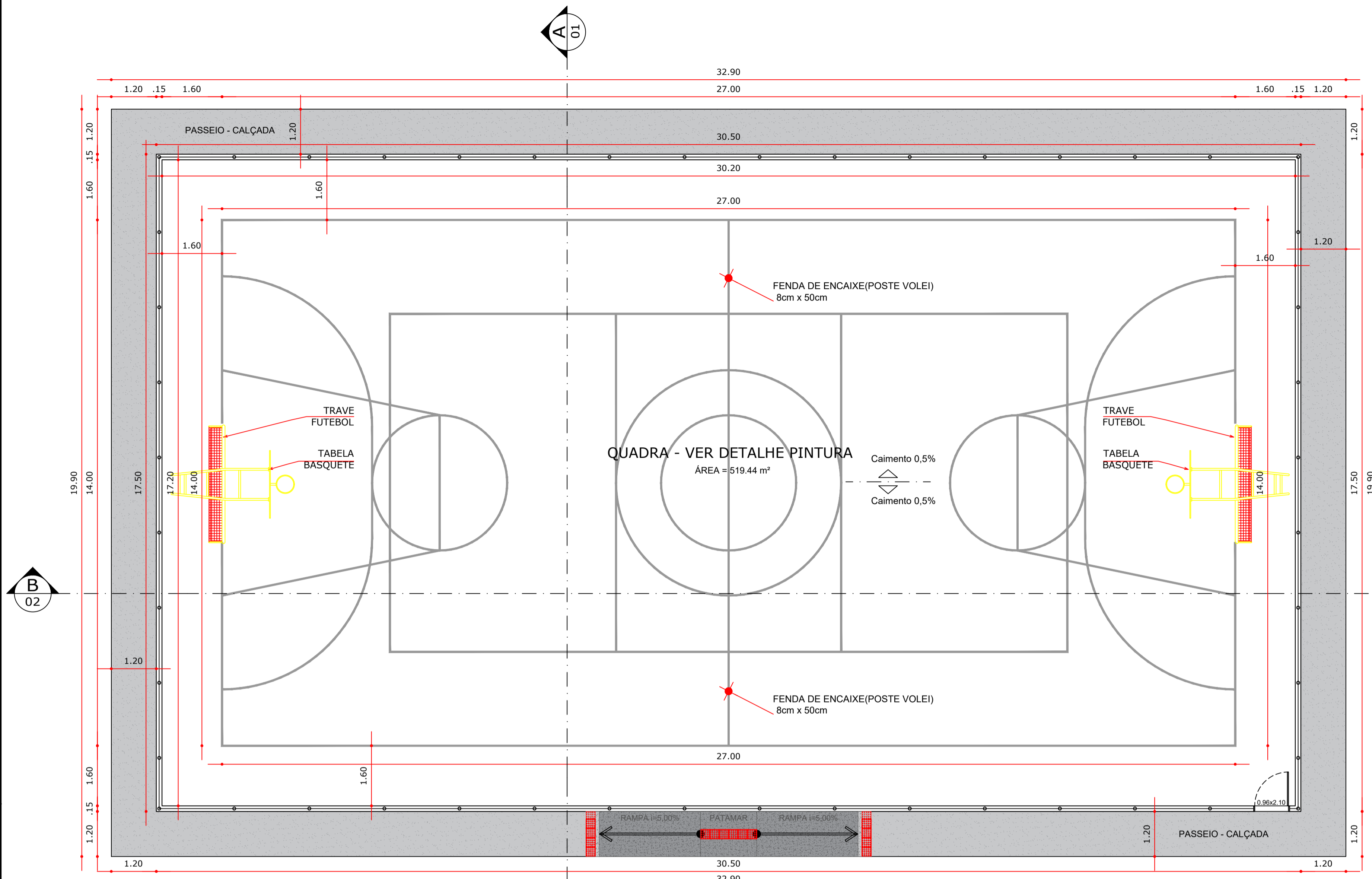
PLANTA DE SITUAÇÃO ESCALA 1:75
